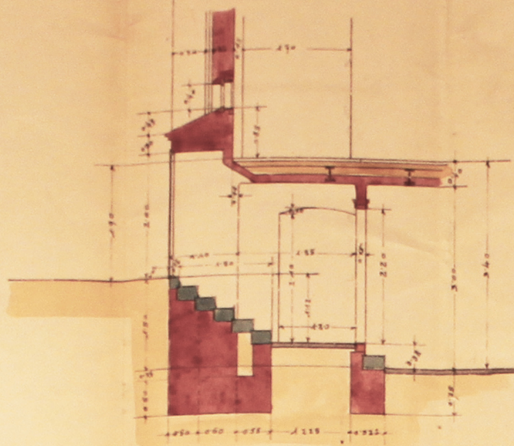
·A-B· METSZET·
